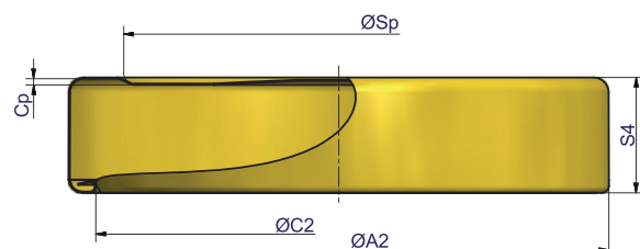
Verschlussstyp DOB
